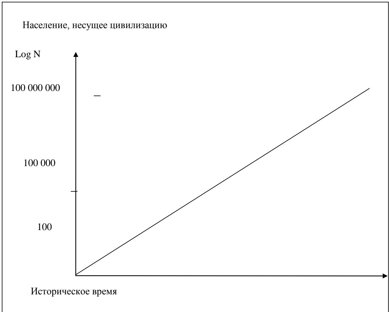
Рис. 1. Рост сложности цивилизаций, выраженный как численность несущих их обществ
